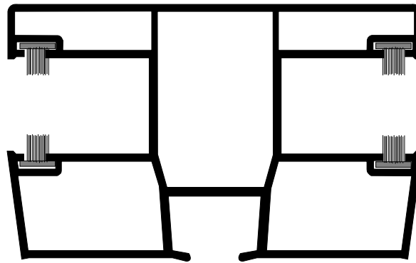
Art. Nr. 939 -B4 - 4 Bürsten - zweiseitig -
